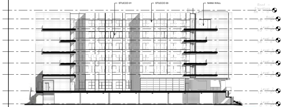
② LONGITUDINAL SECT 02 1/16" = 1'-0"
