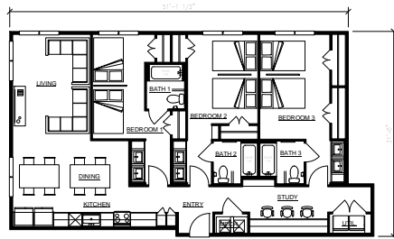
11 UNIT F4 1/8"=1'-0" 1591 SF
