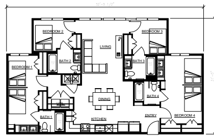
9 UNIT F2B 1/8"=1'-0" 1483 SF
