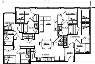
8 UNIT F2A 1/8"=1'-0" 1811 SF
