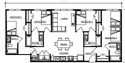
6 UNIT E1A 1/8"=1'-0" 1335 SF
