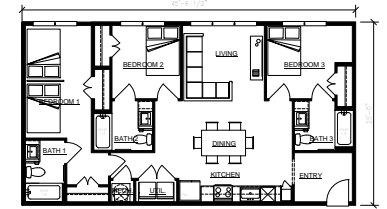
3 UNIT D2 1/8"=1'-0" 1139 SF
