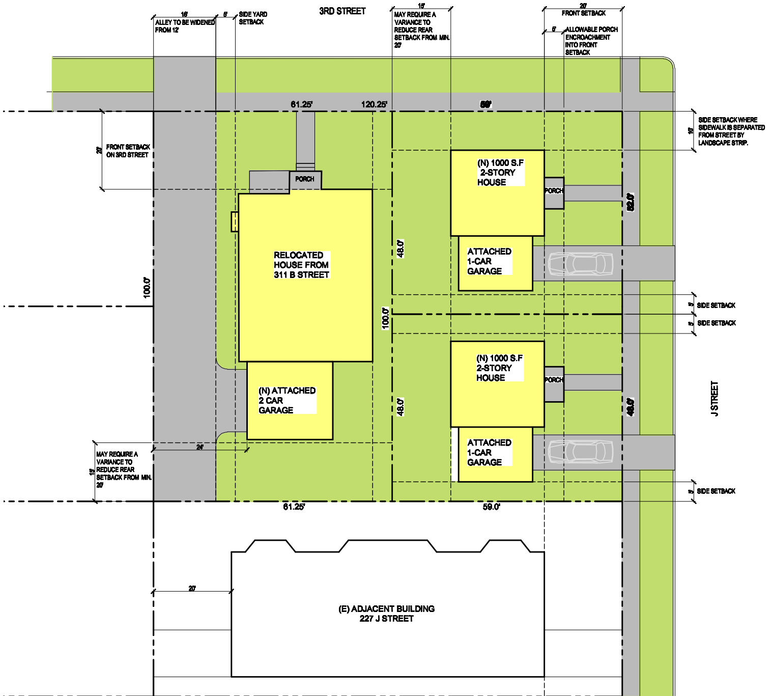
SITE PLAN - OPTION C
